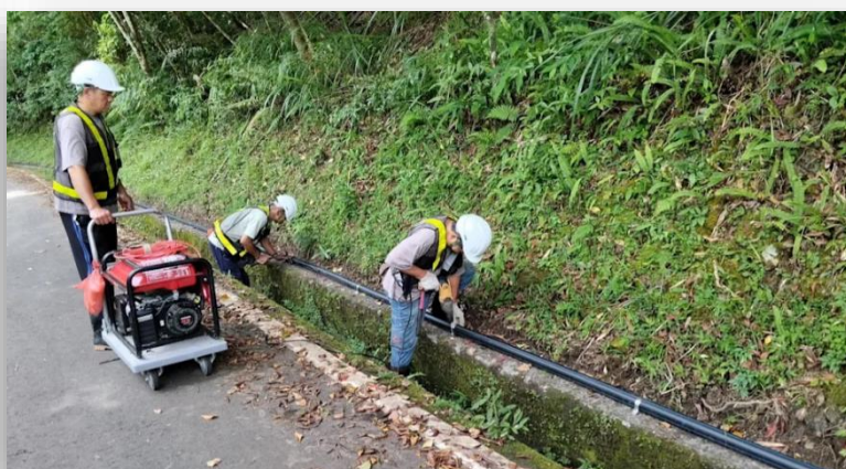
圖 二十九、福山里卡拉模基採用抗壓、耐震及韌性佳的 HDPE 水管
